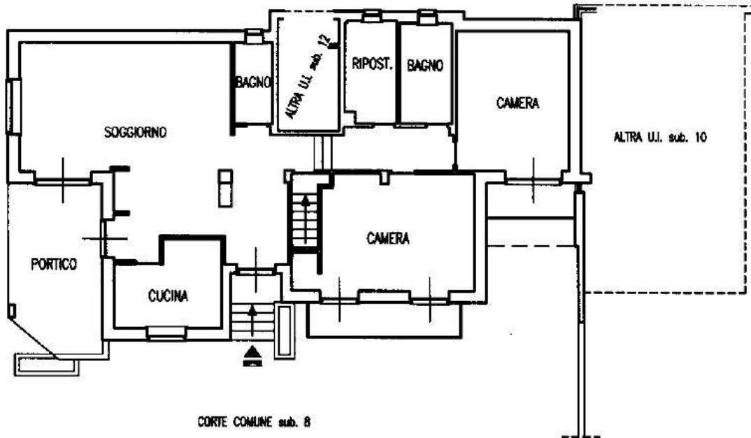
Pianta Piano Terreno h. 2,90
